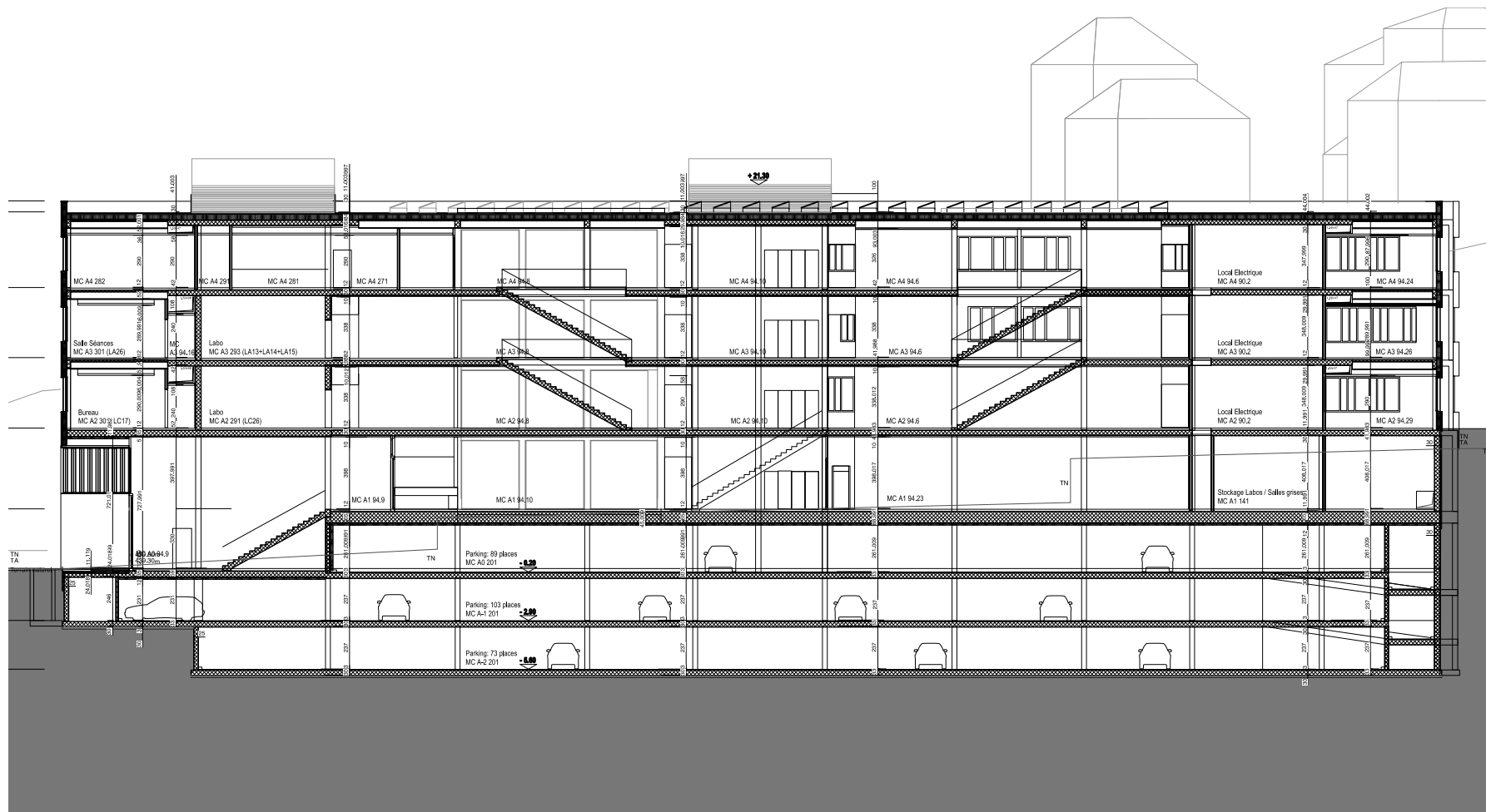
Coupe longitudinale
